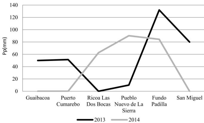
Fig. 5. Precipitación 2013-2014 Embalse El Isiro. Fuente: Instituto Nacional de Meteorología e Hidrología (INAMEH)
