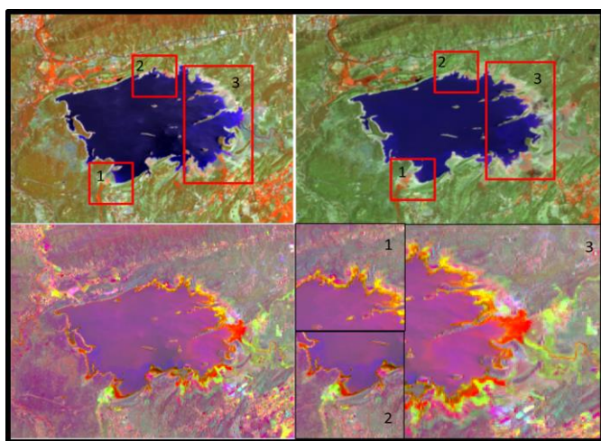
Fig. 3. MAD, 2013-2014 Imagen Landsat 8-OLI, en los recuadros puede observarse que el geoalgoritmo coloca de color rojo los mayores cambios y de color amarillo los cambios medios.
